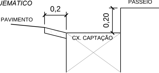
CORTE TRANSVERSAL -A-A ESQUEMÁTICO
