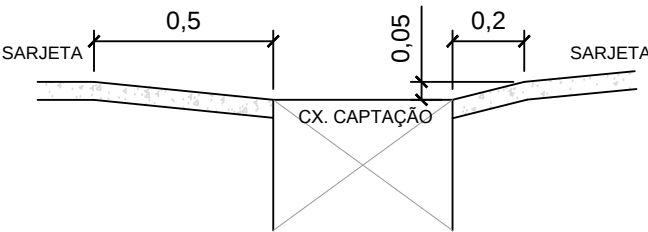
CORTE LONGITUDINAL -B-B ESQUEMÁTICO
