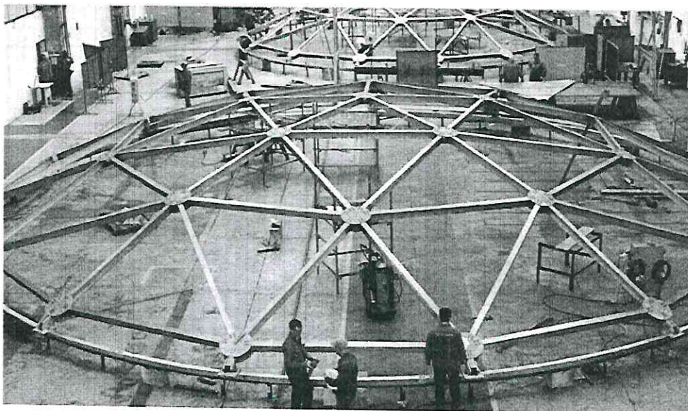
FABRICAÇÃO E PRÉ-MONTAGEM DOS TETOS TIPO DOMO GEODÉSICOS NA FÁBRICA DA TEQUALY
