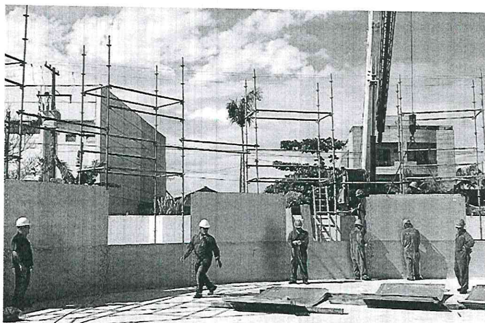
MONTAGEM DO COSTADO EM CAMPO A TEQUALY TEM TODOS OS EQUIPAMENTOS NECESSÁRIOS PARA A MONTAGEM
