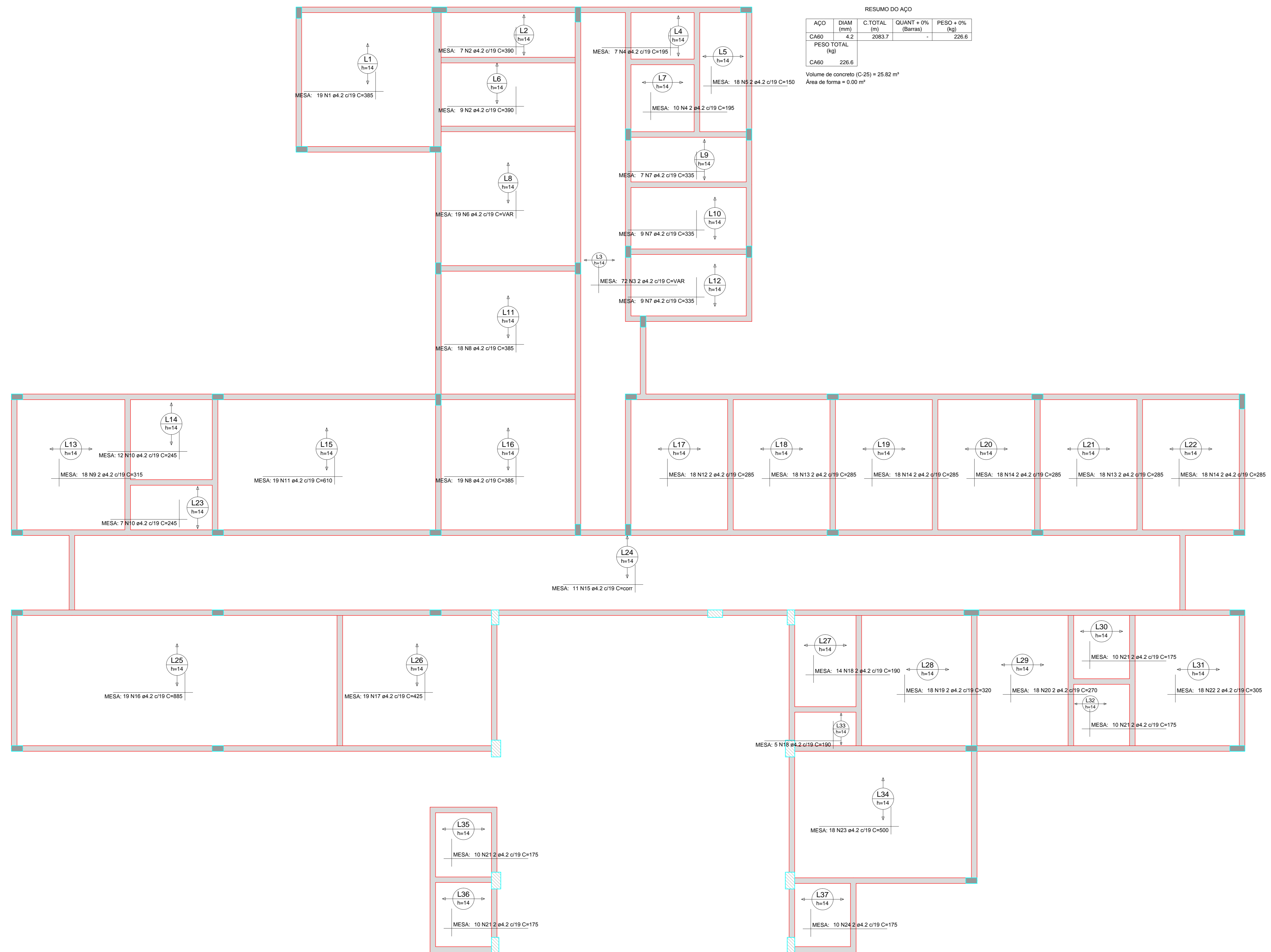
Armação positiva das lajes do pavimento Terreo (Eixo X) escala 1:50
