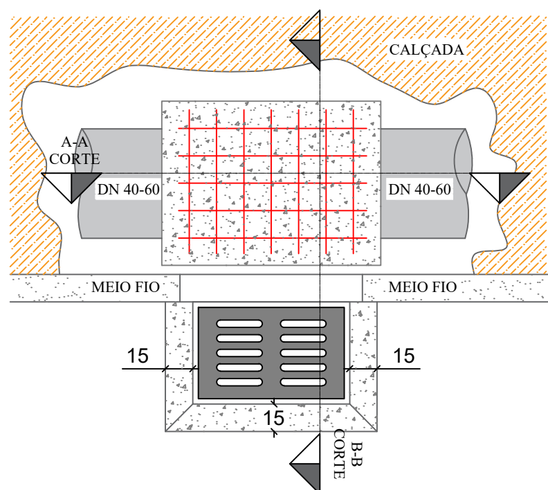
PLANTA BAIXA GRELHA DE CONCRETO
