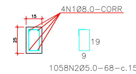
DET. VIGA BALDRAME (15x25)(58.6m) ESCALA 1:20
