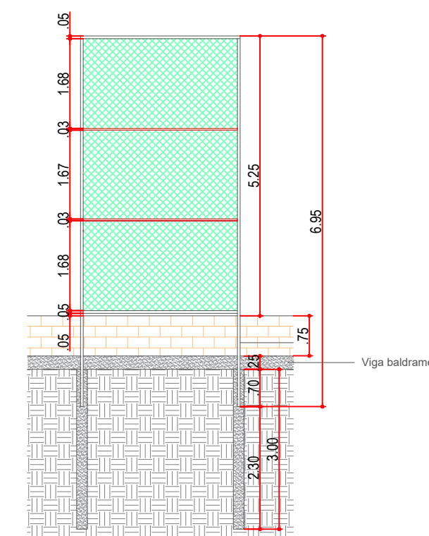
DETALHE FUNDAÇÃO VISTA B ESC: 1/100
