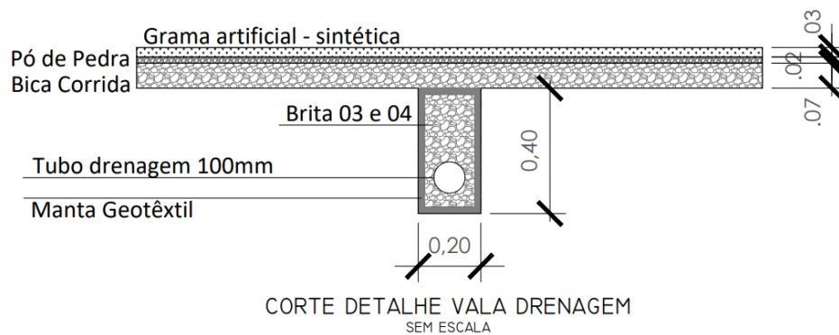
Figura 05 – Detalhe de instalação Drenagem (Fonte: Autora/2021)
