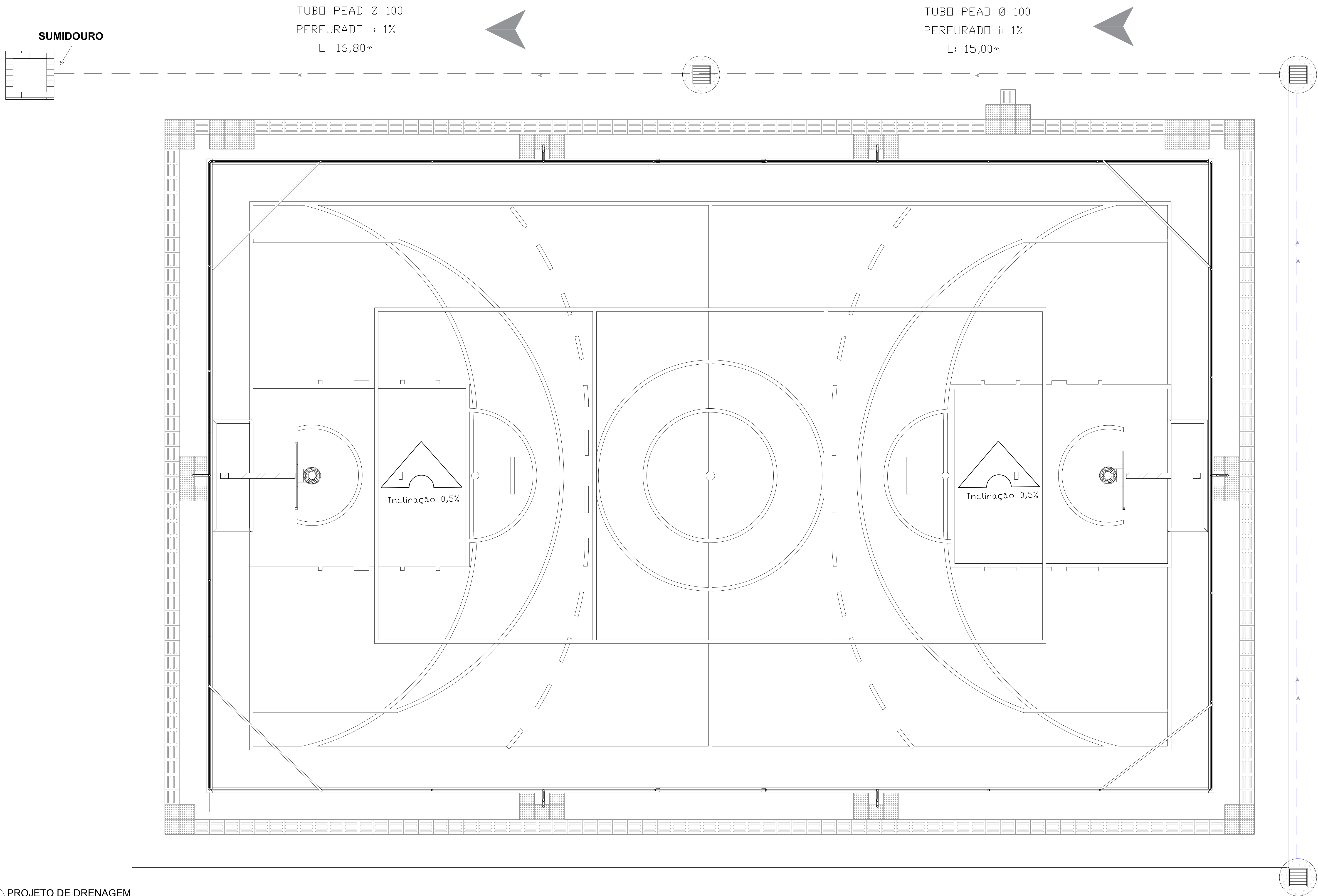
01 PROJETO DE DRENAGEM ESC. 1:125
