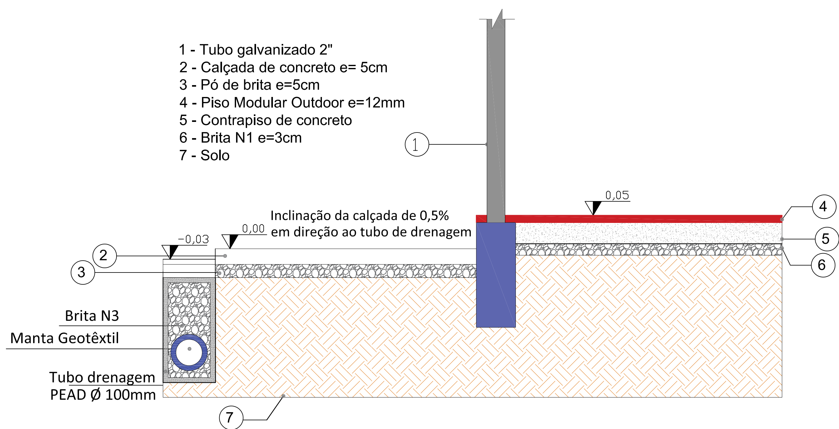
02 DETALHE DE PISOS S/ ESCALA
