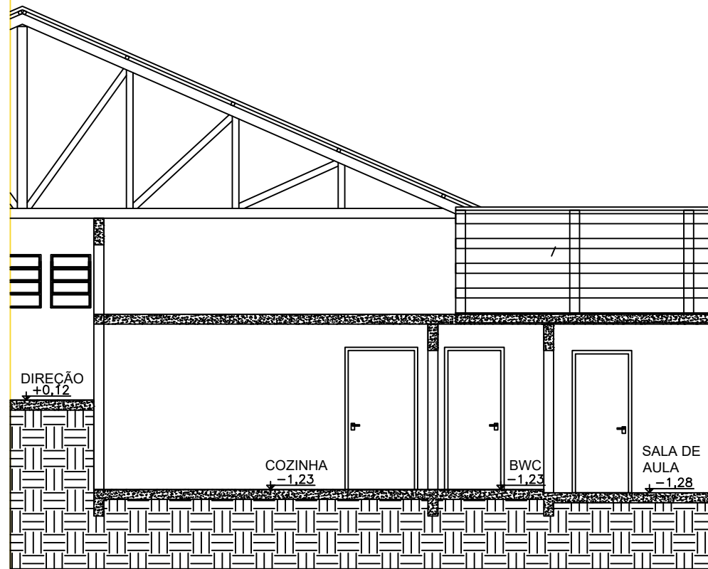
CORTE AA - REFORMA Esc: 1/50
