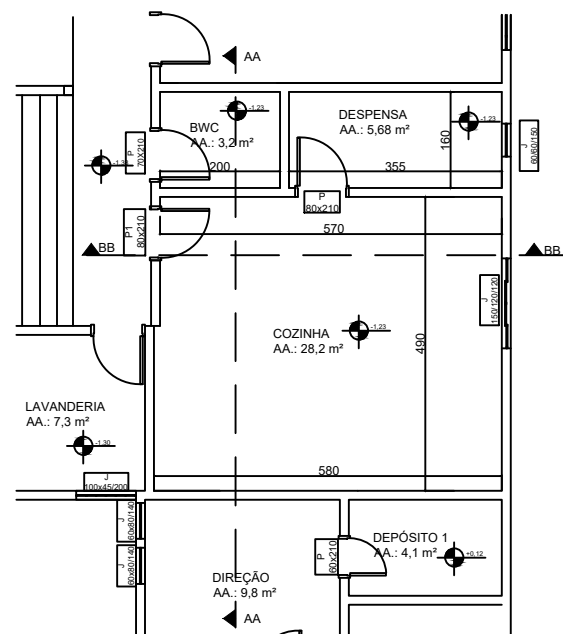
PROJETO REFORMA Esc: 1/50
