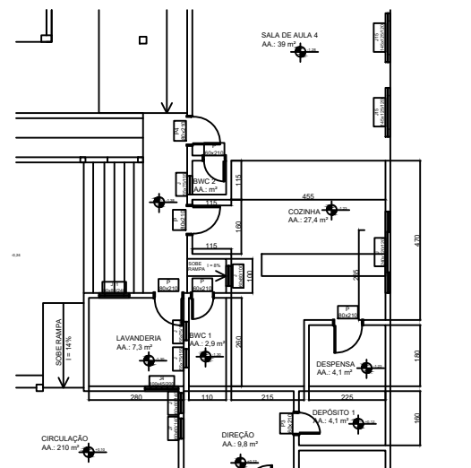
EDIFICAÇÃO ATUAL Esc: 1/50
