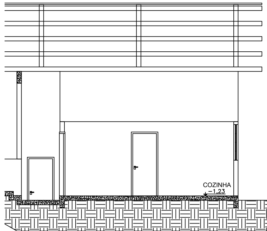
CORTE BB - REFORMA Esc: 1/50
