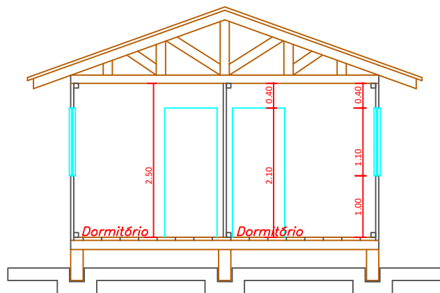
Corte AB Esc.:1/50
