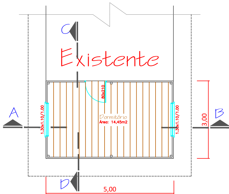
Planta Baixa - Ampliação Esc.:1/50
