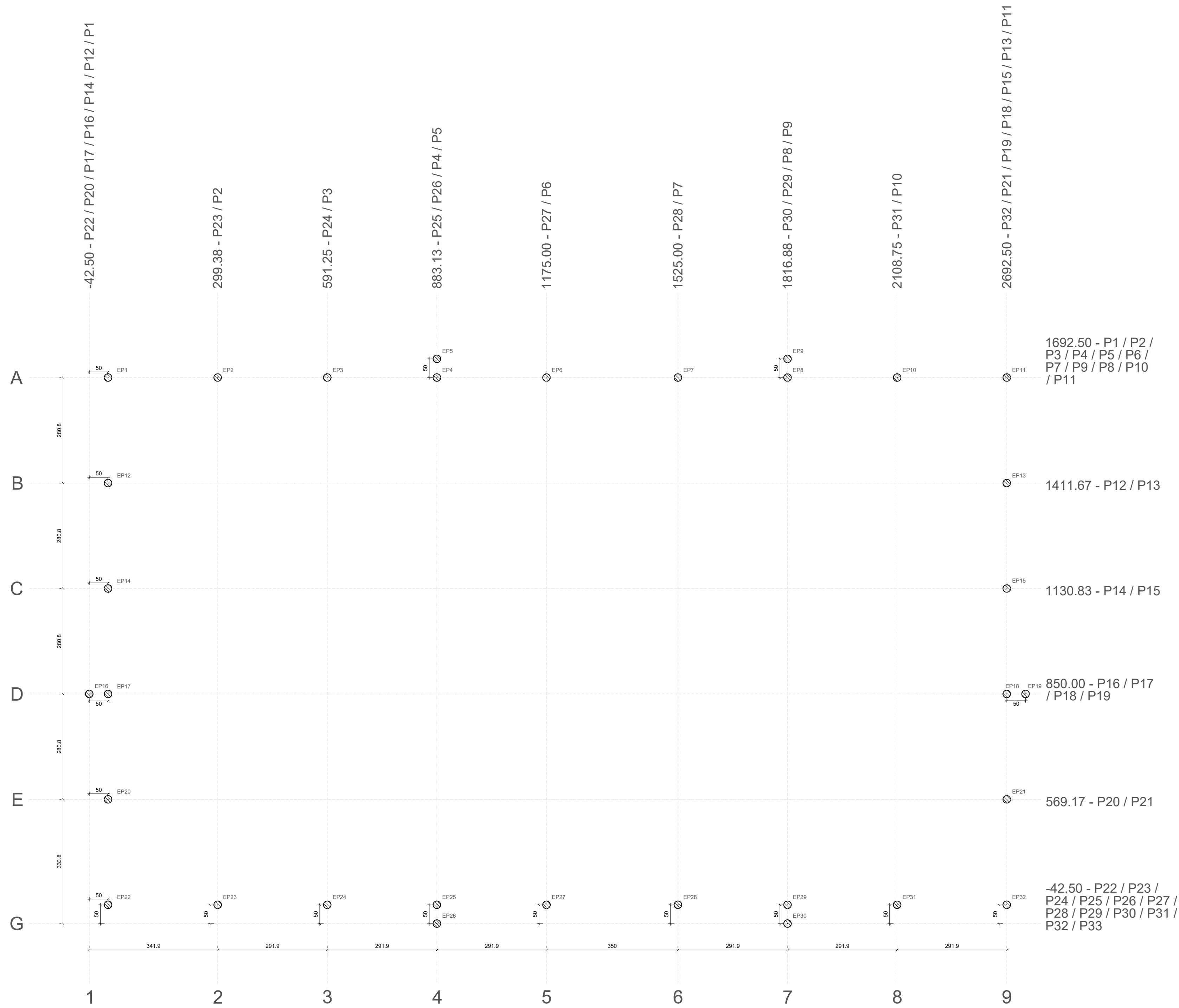
Planta de cargas escala 1:50
