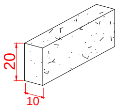
detalhe viga de travamento em concreto FCK= 20MPa
