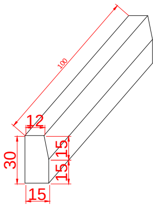
detalhe Meio-fio em concreto FCK= 15MPa
