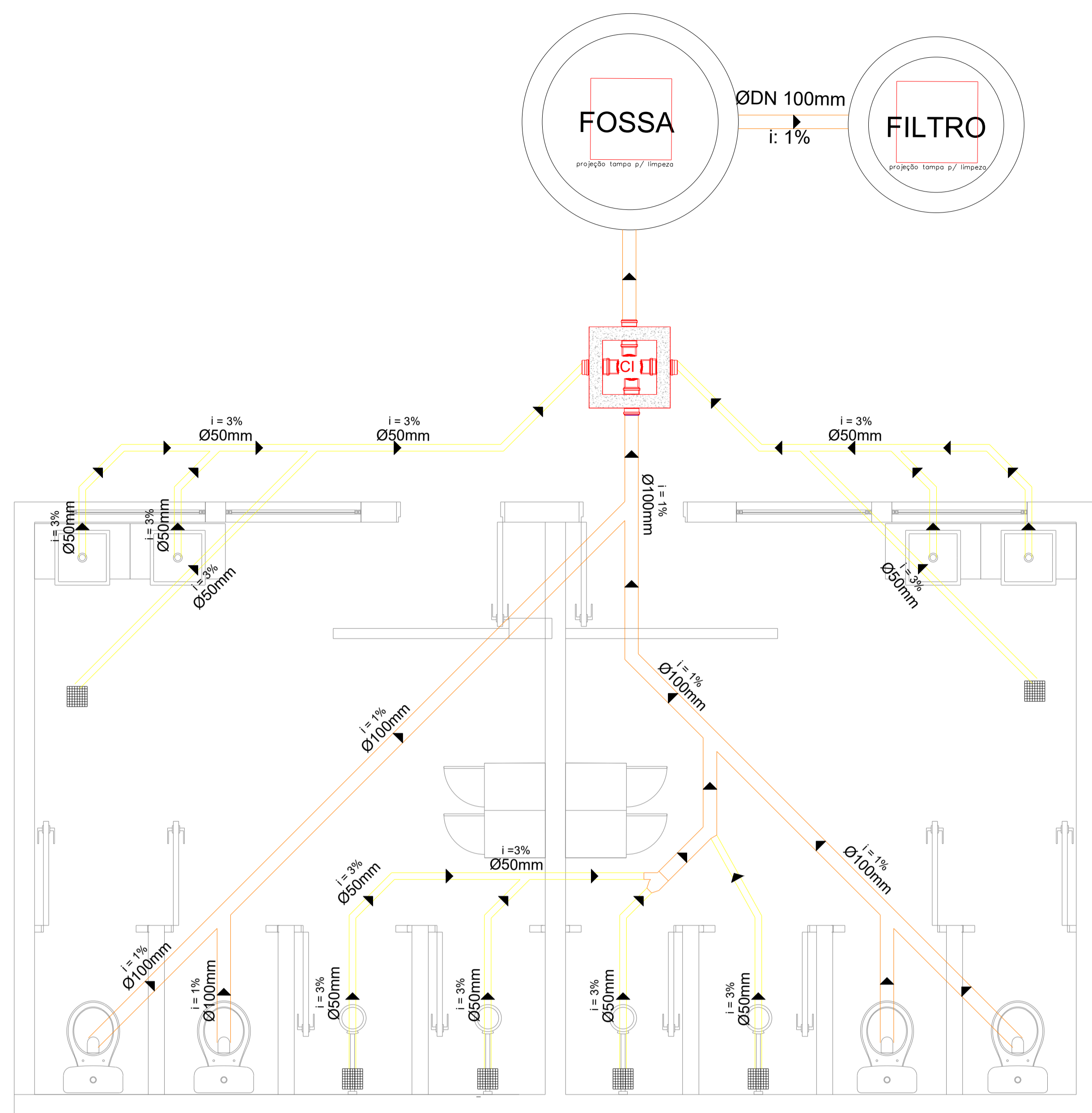
PLANTA BAIXA INSTALAÇÕES SANITÁRIAS 1/25
