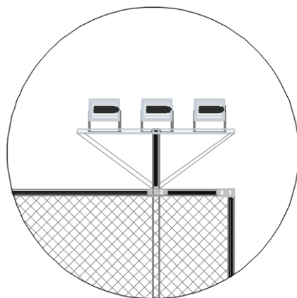
Figura 10 – Detalhe de instalação dos refletores (Fonte: Autor/2024)
