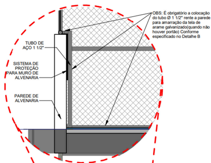
Figura 08 – Detalhe da fixação das telas (Fonte: Autor/2024)
