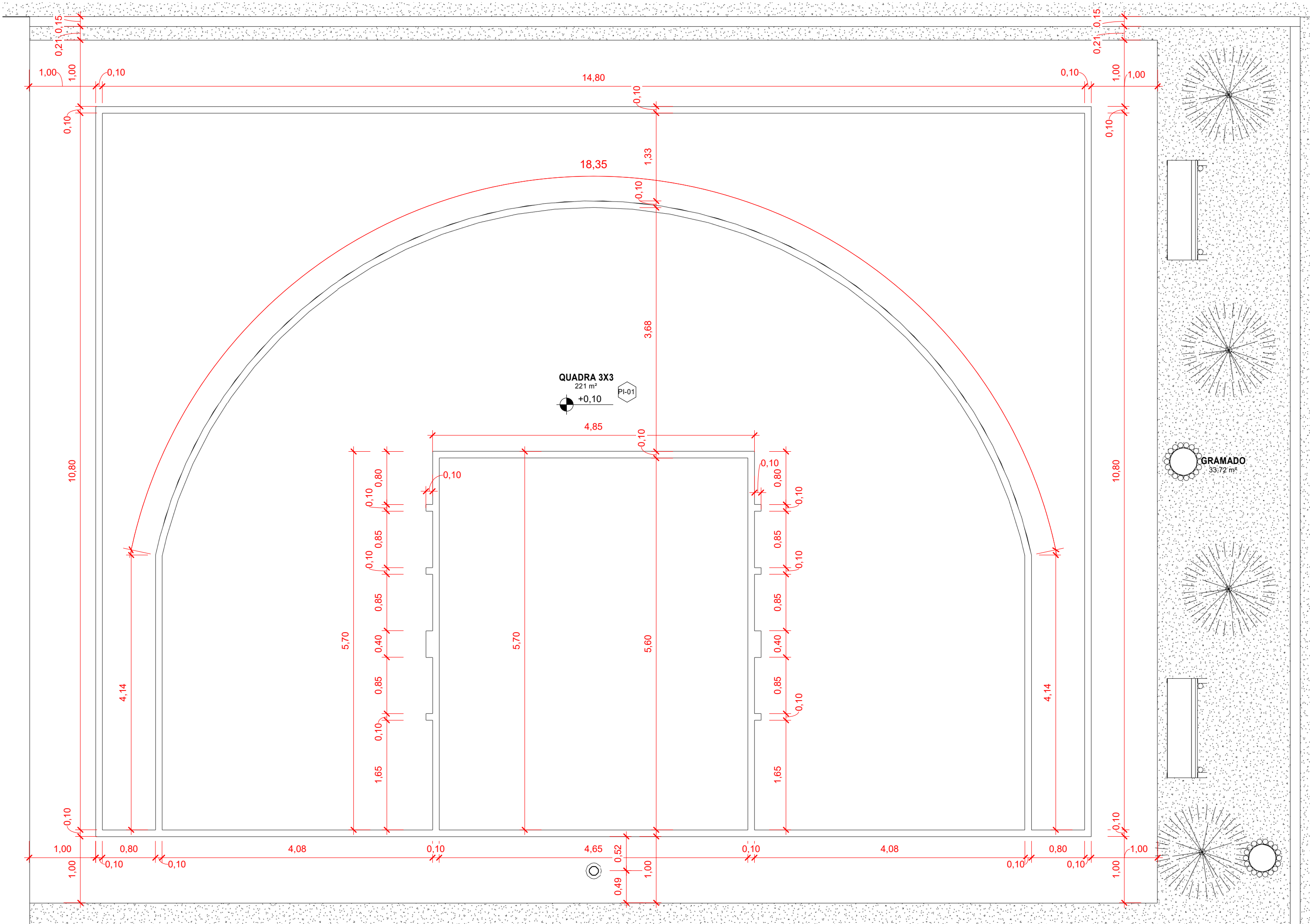
1 Planta Baixa - Quadra 3x3 Executivo 1 : 50
