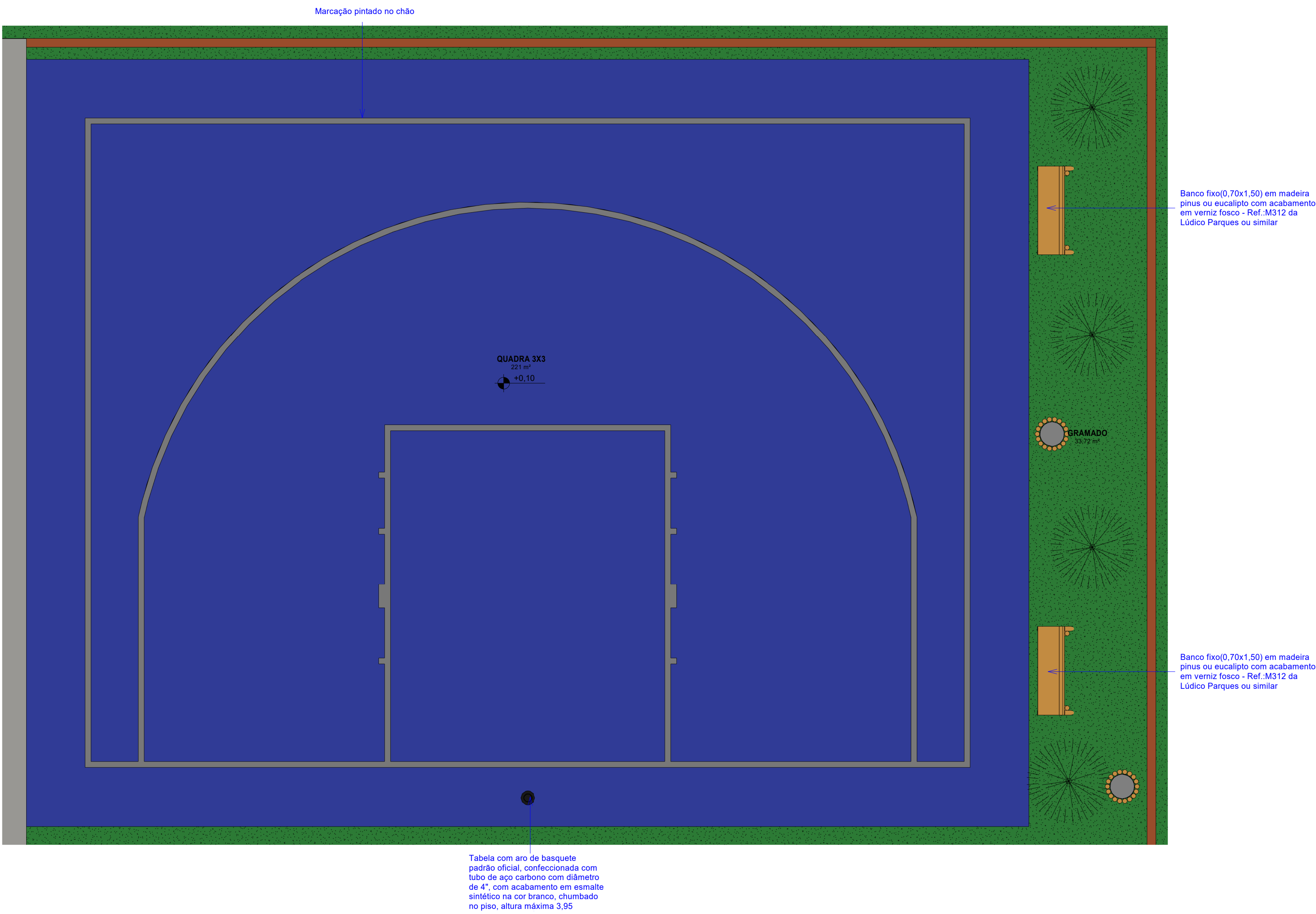
2 Planta Baixa - Quadra 3x3 Layout 1 : 50
