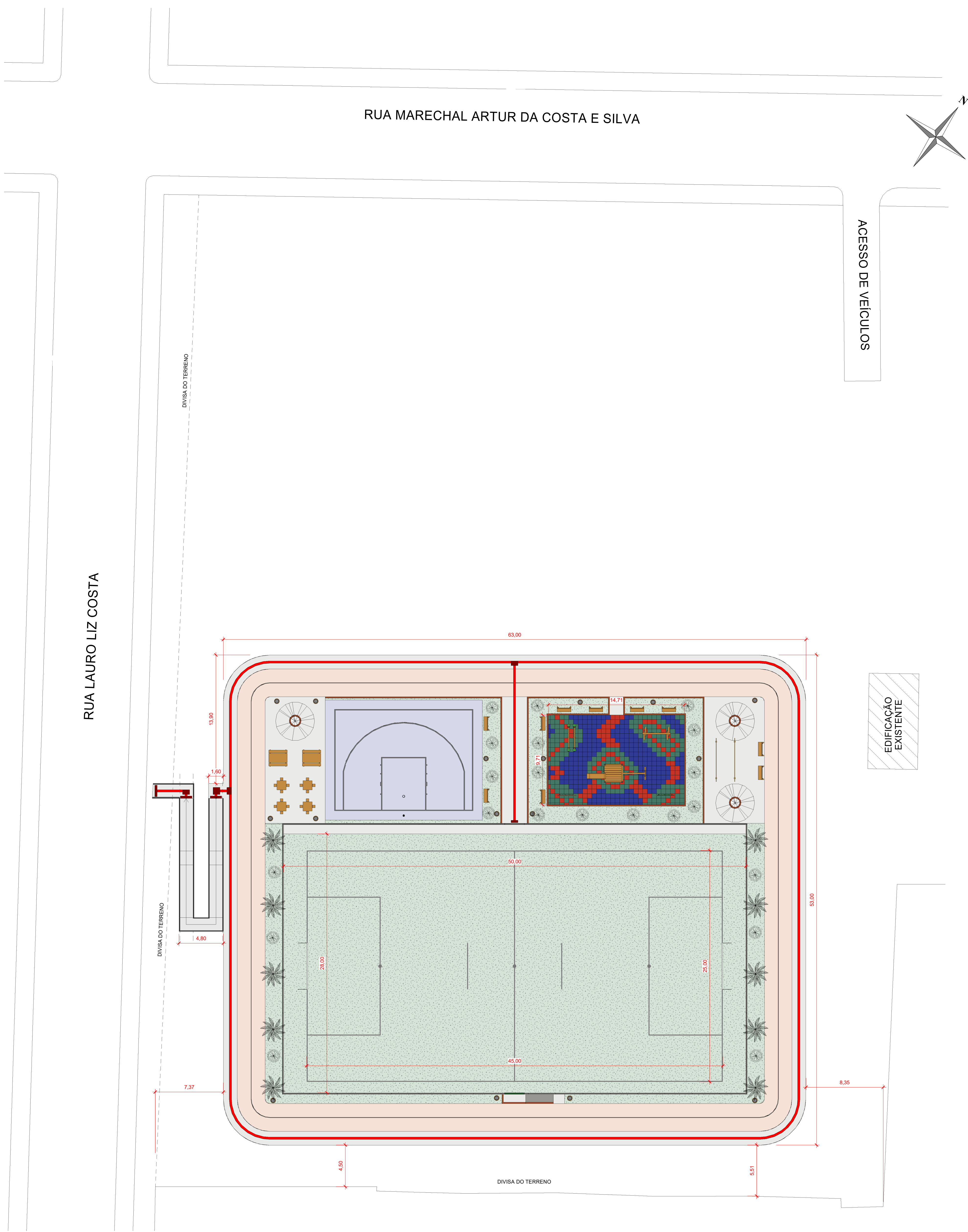
1 PLANTA DE LOCAÇÃO 1 : 200
