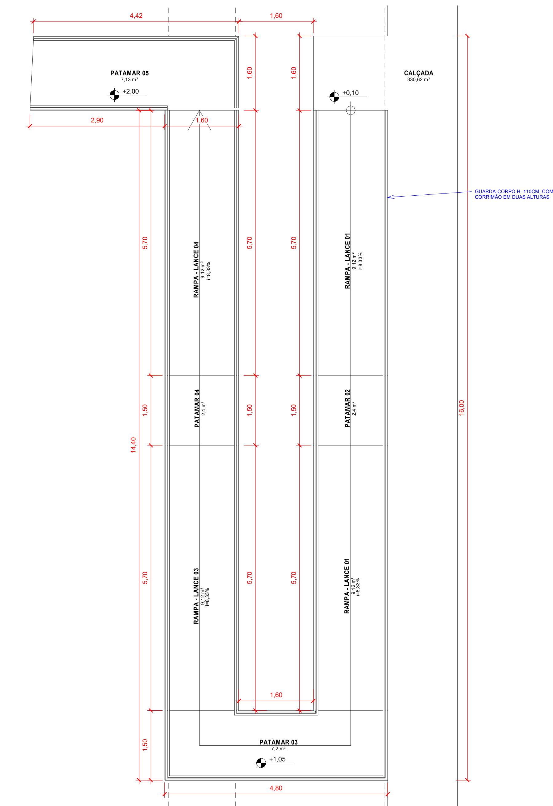
2 Planta Baixa - Rampa 1 : 50
