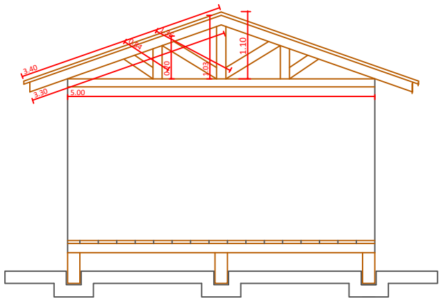
Corte CD
