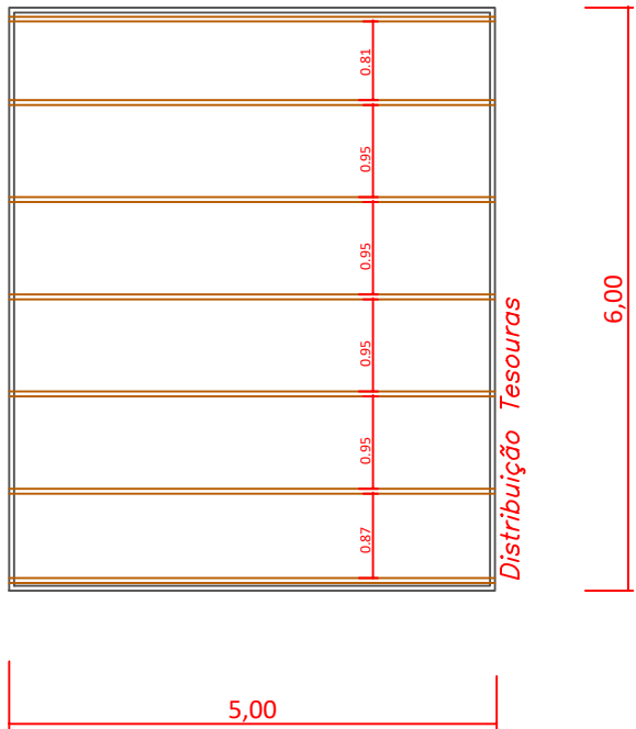
Detalhamento Telhado
