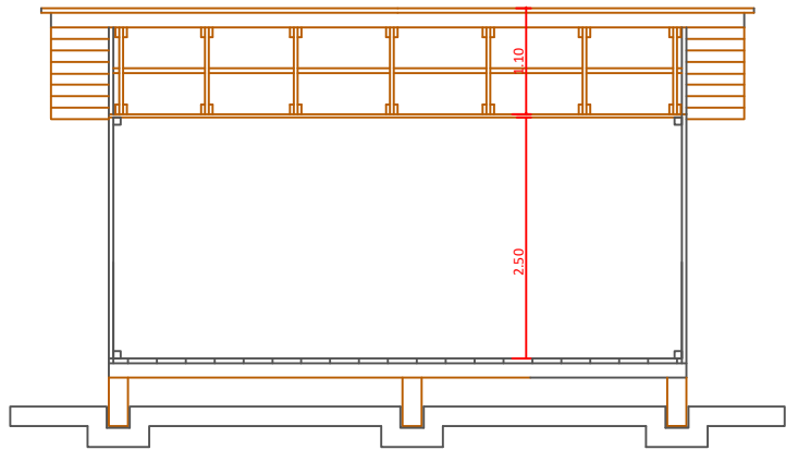
Corte CD
