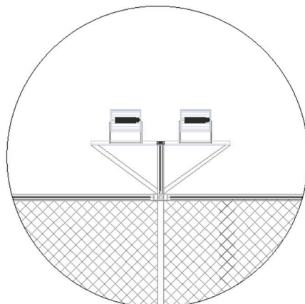
Figura 09 – Detalhe de instalação dos refletores (Fonte: Autor/2023)
