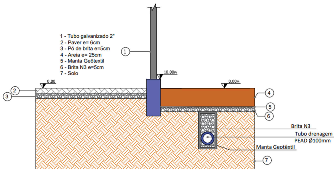
Figura 04 – Detalhe do tubo de drenagem (Fonte: Autor/2023)
