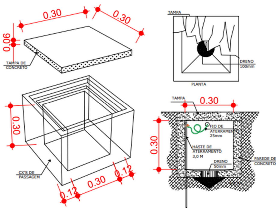
Figura 08 – Detalhe de instalação da caixa de aterramento (Fonte: Autor/2024)
