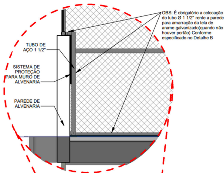
Figura 07 – Detalhe da fixação das telas (Fonte: Autor/2024)
