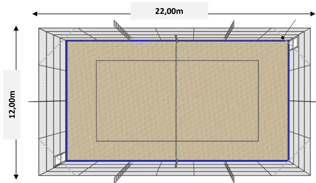
Figura 02 – Dimensões do Quadra de Areia (Fonte: Autor/2023)
