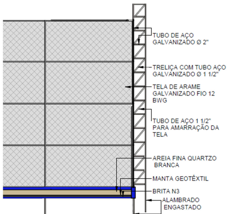
Figura 05 – Detalhe de instalação do alambrado (Fonte: Autor/2023)
