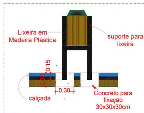
Figura 11 - Detalhe Ilustrativo Fixação da lixeira (Fonte: Autor/2025)
