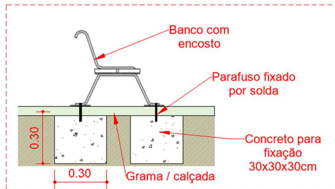
Figura 10 - Detalhe ilustrativo fixação do banco (Fonte: Autor/2025)
