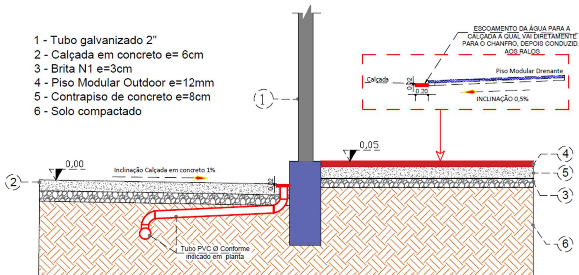
Figura 4 – Detalhe de instalação da drenagem (Fonte: Autor/2025)
