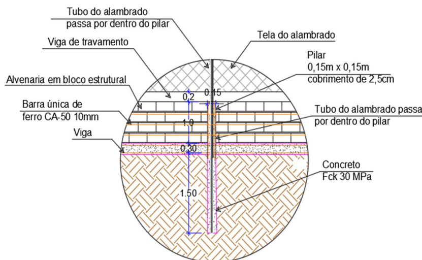
Figura 5 – Detalhamento de estaca (Fonte: Autor/2025)
