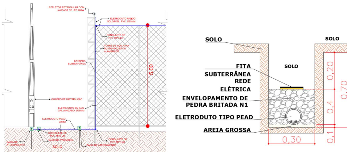
Figura 13 - Detalhes da elétrica (Fonte: Autor/2025)
