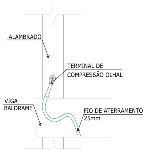
Figura 14 – Detalhe de aterramento da quadra (Fonte: Autor/2025)
