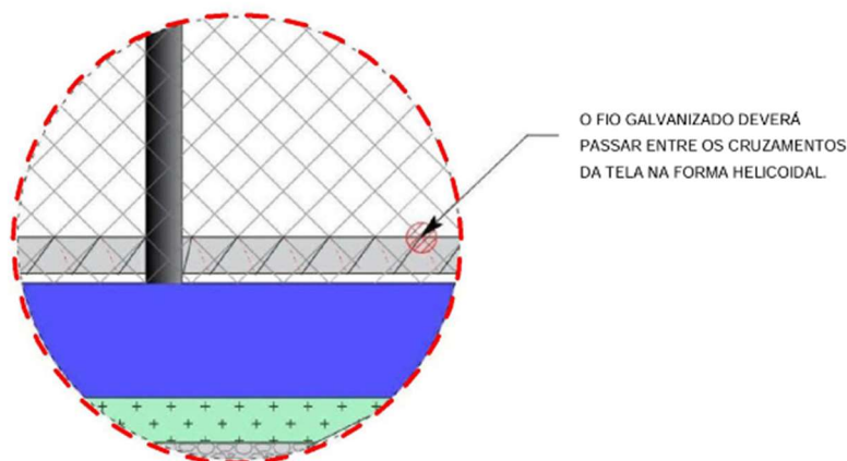
Figura 7 – Detalhe da fixação das telas (Fonte: Autor/2025)
