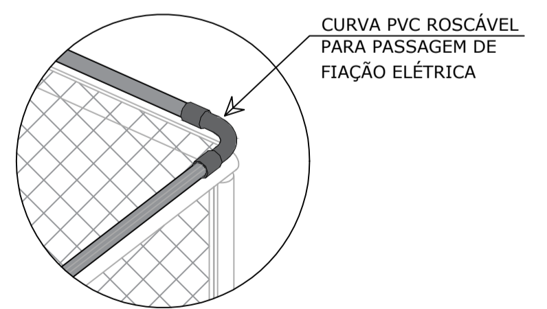
10 DETALHE CURVA PVC ROSCÁVEL S/ESCALA
