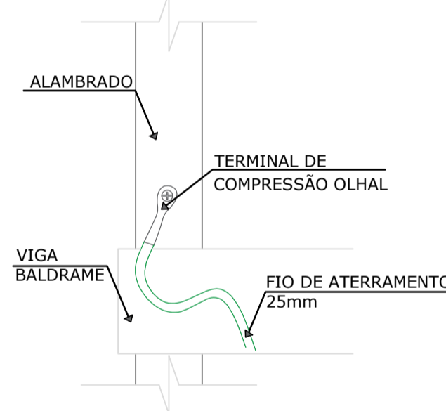
9 DETALHE TERMINAL OLHAL S/ESCALA
