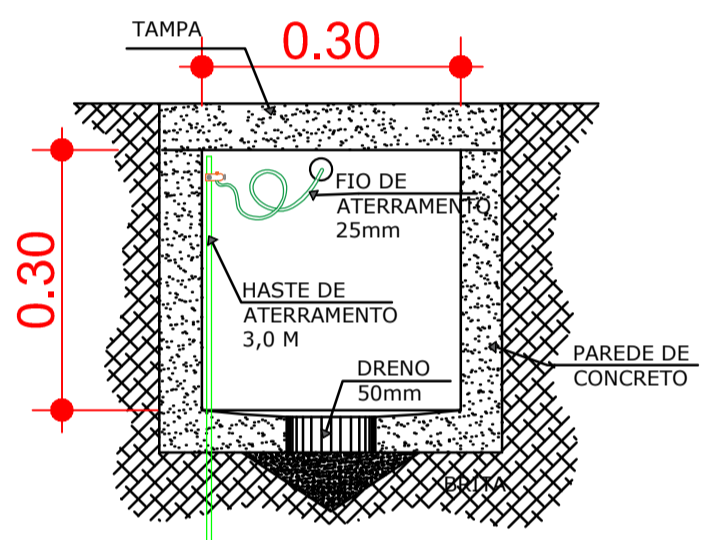
7 CORTE CAIXA DE PASSAGEM S/ESCALA
