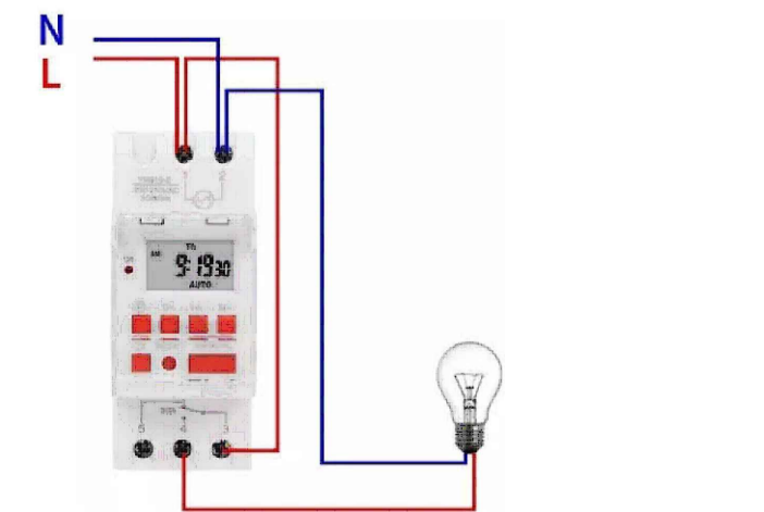
12 DETALHE TIMER S/ESCALA
