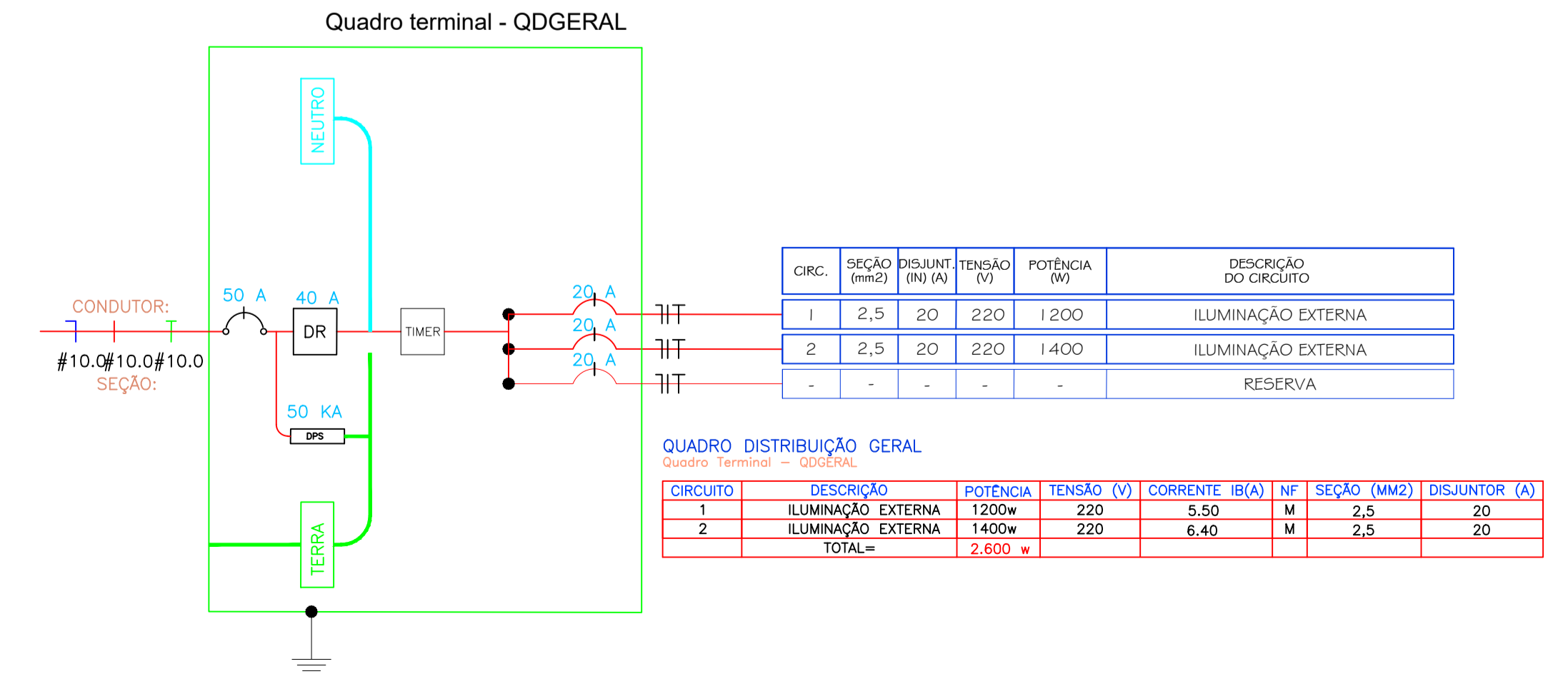
14 DIAGRAMA UNIFILAR S/ESCALA
