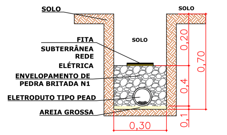
11 CORTE FITA DE IDENTIFICAÇÃO REDE ELÉTRICA S/ESCALA
