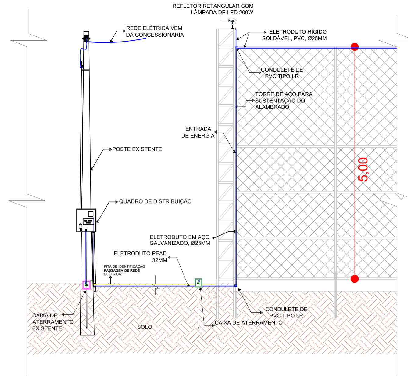
3 DETALHAMENTO ALAMBRADO S/ESCALA
