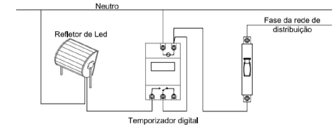
5 ESQUEMA DE INSTALAÇÃO REFLETORES S/ESCALA
