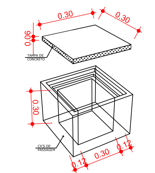
6 PERSPECTIVA CAIXA DE PASSAGEM S/ESCALA
