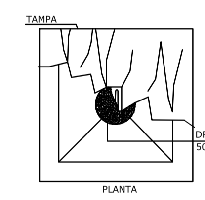
8 PLANTA CAIXA DE PASSAGEM S/ESCALA
