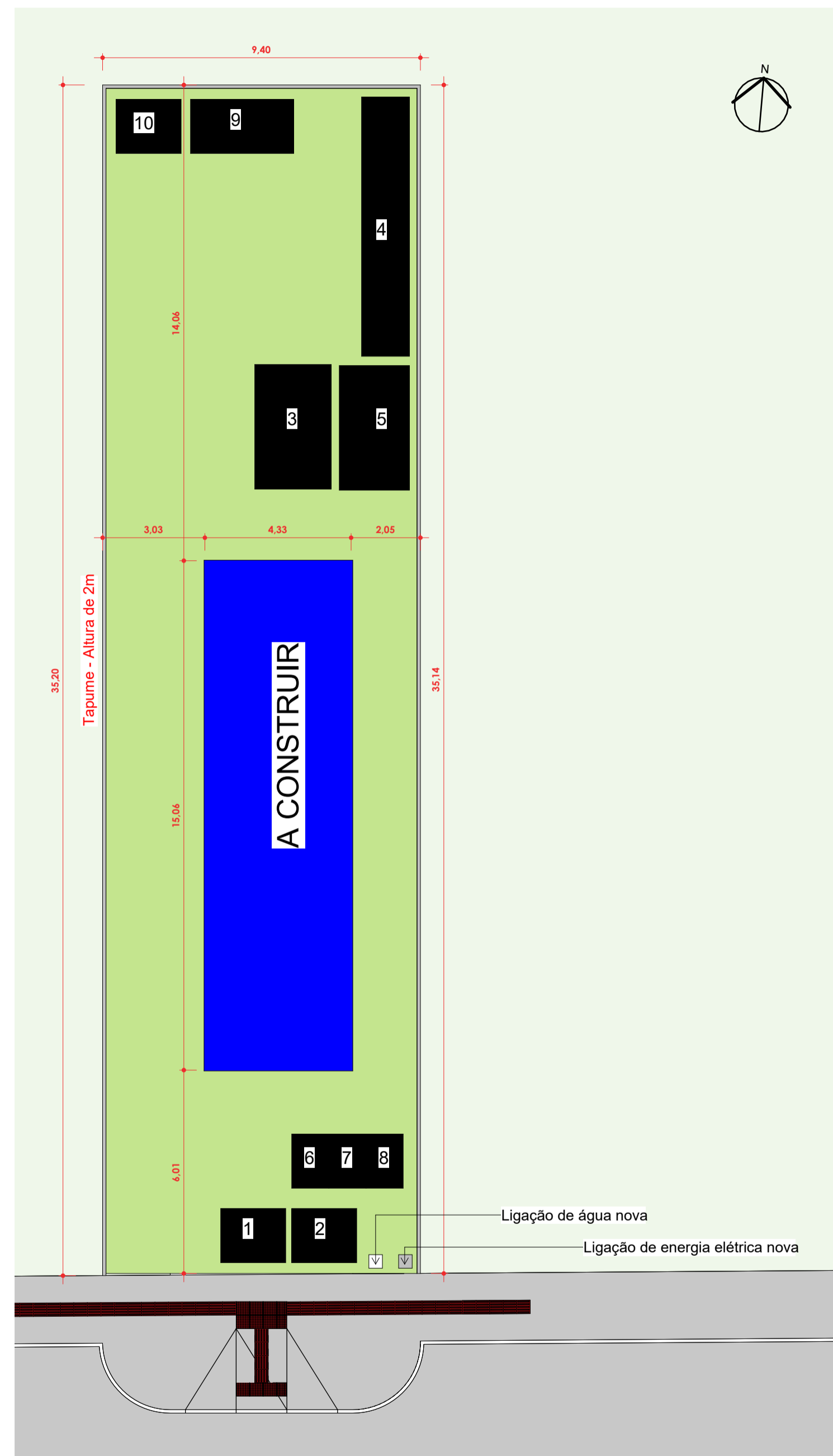
1 LAYOUT CANTEIRO DE OBRAS 1 : 125
