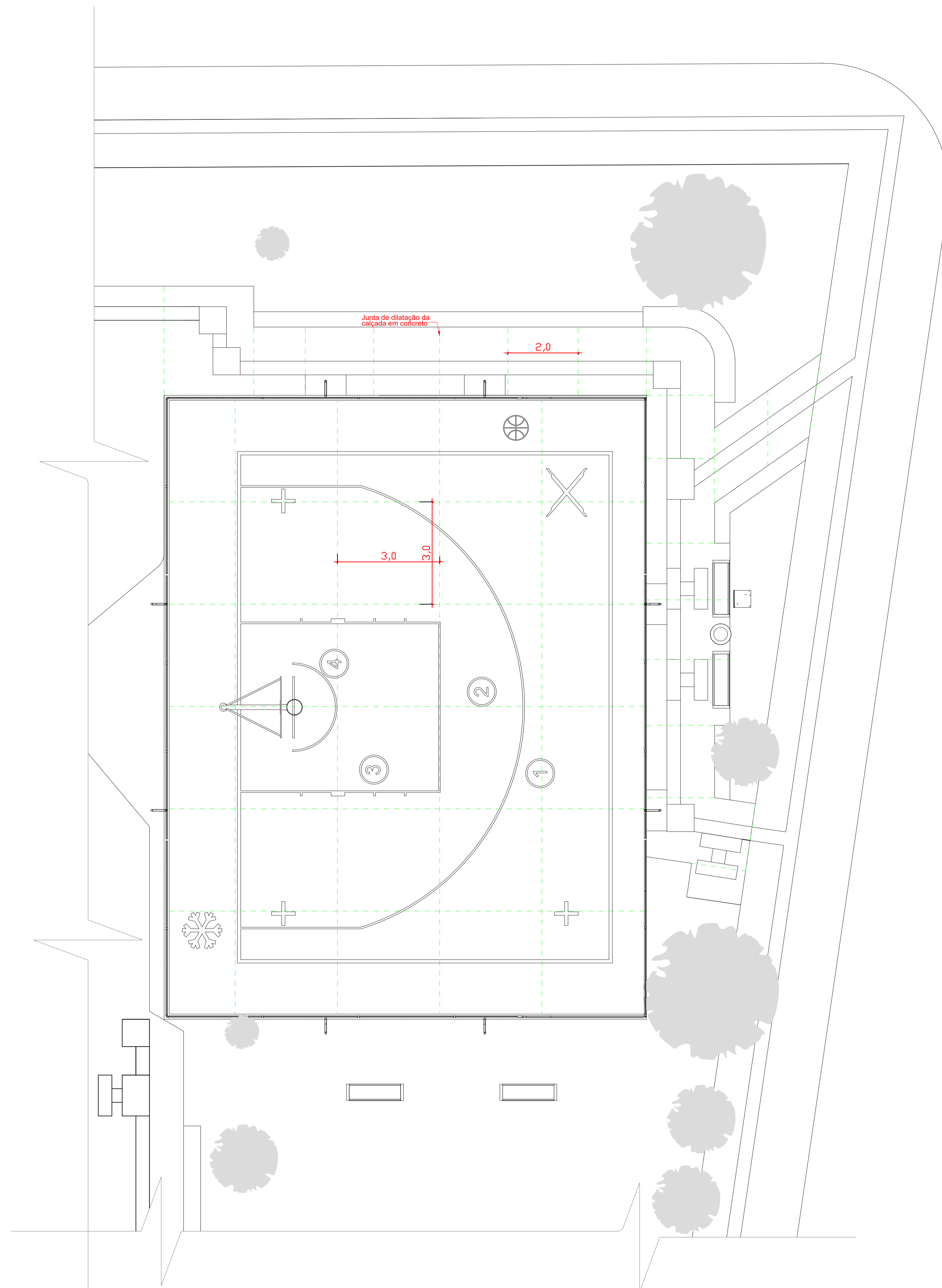
PLANTA DE JUNTAS DE DILATAÇÃO Escala 1:50
