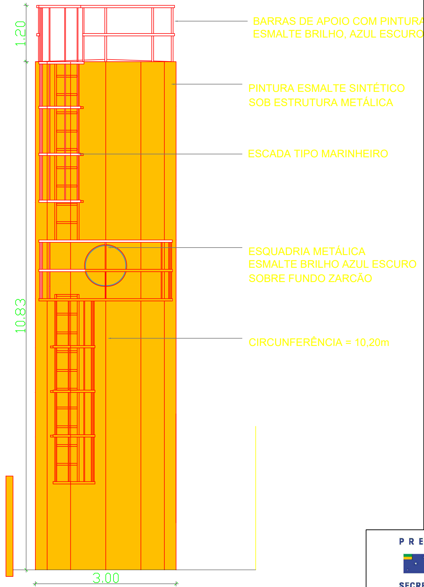
PINTURA CAIXA D'ÁGUA ESC: 1/50
