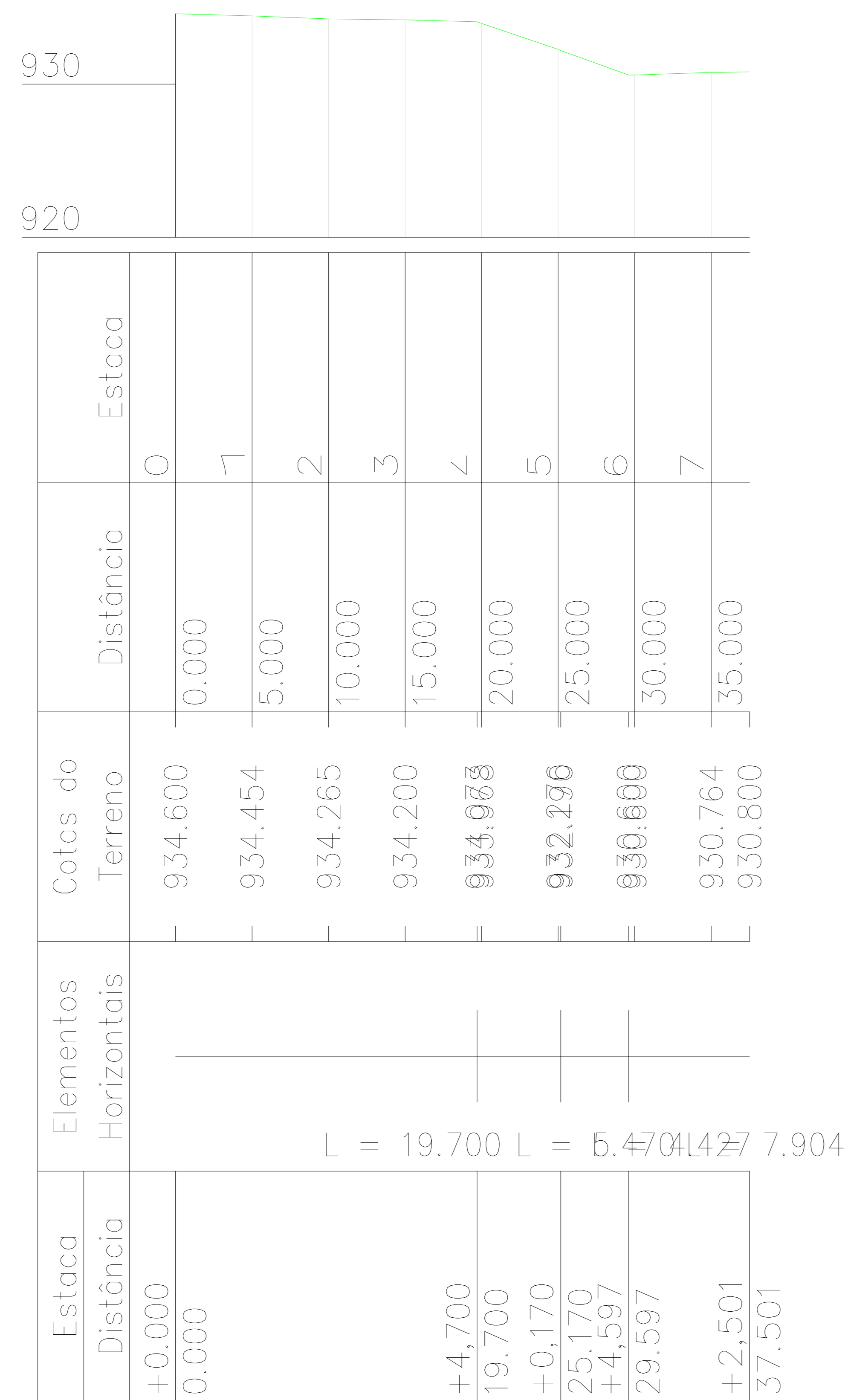
1 PERFIL LONGITUDINAL - RAMPA SEM ESCALA
