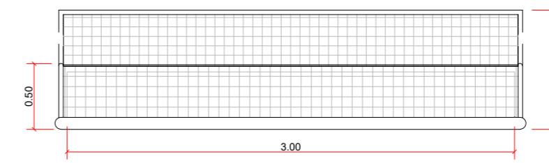
01 BALIZA FUTEBOL ESC. 1:25
