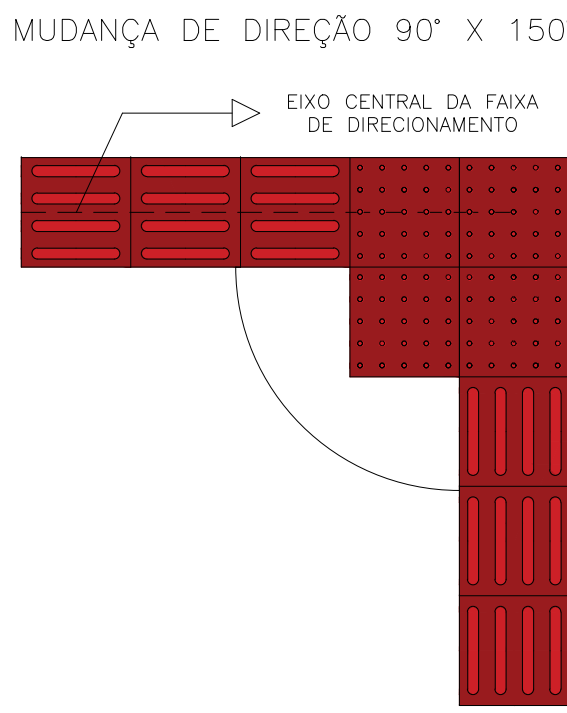
4 DET 01 Escala 1/50
