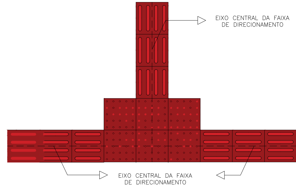
5 DET 02 Escala 1/50
