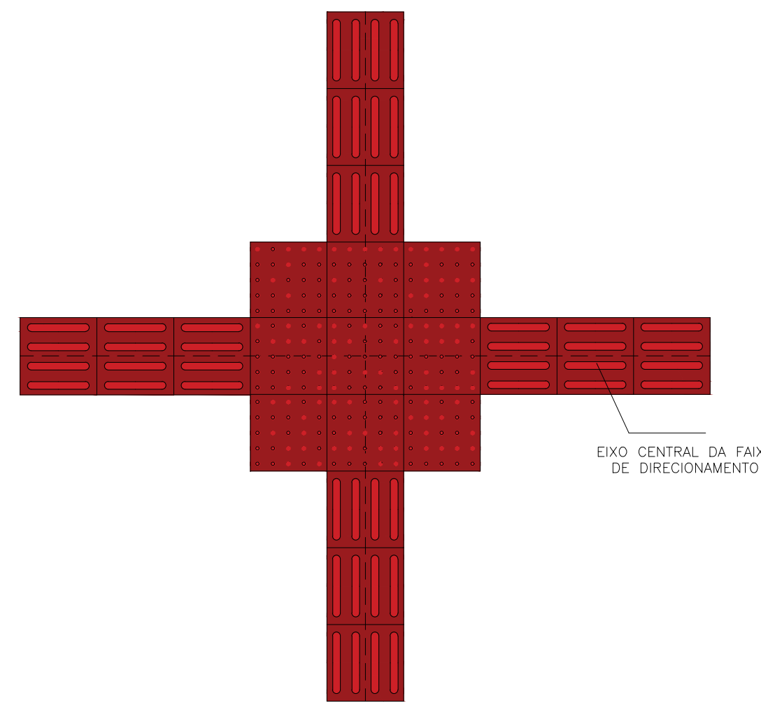
6 DET 03 Escala 1/50
