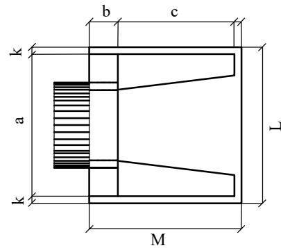
PLANTA NORMAL
