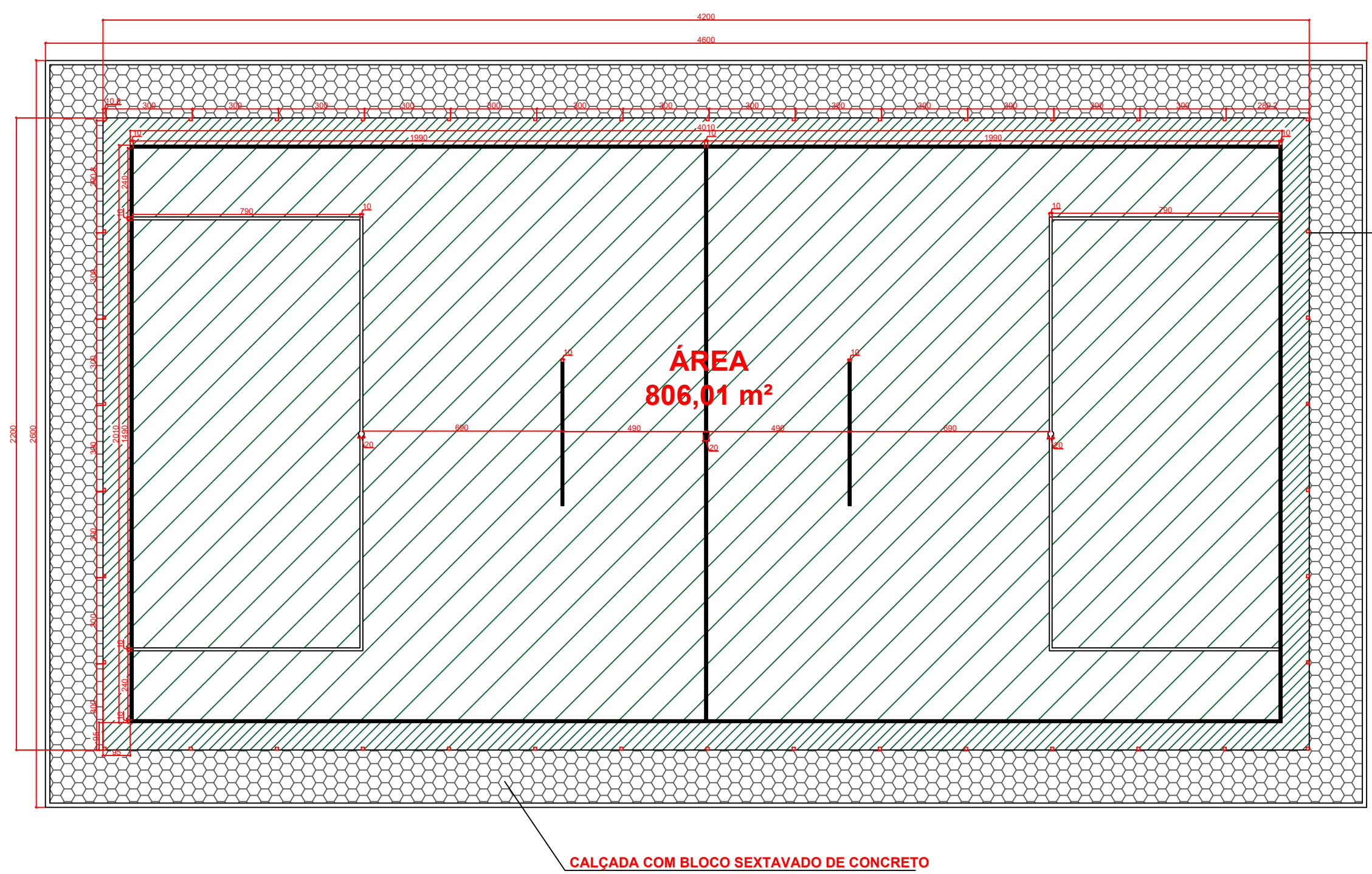
PLANTA DA QUADRA DE GRAMA SINTÉTICA
