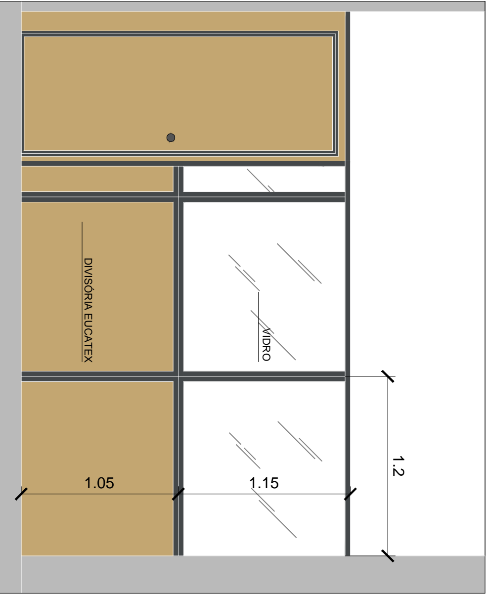
VISTA 1 ESPECIFICAÇÕES DIMENSÕES DIVISÓRIAS EUCATEX ESC.: 1/25
