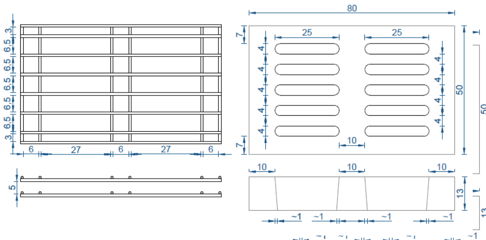
Figura 4 – Grelha modelo
