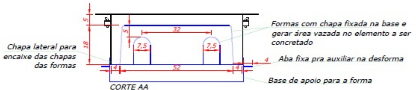
CORTE AA
