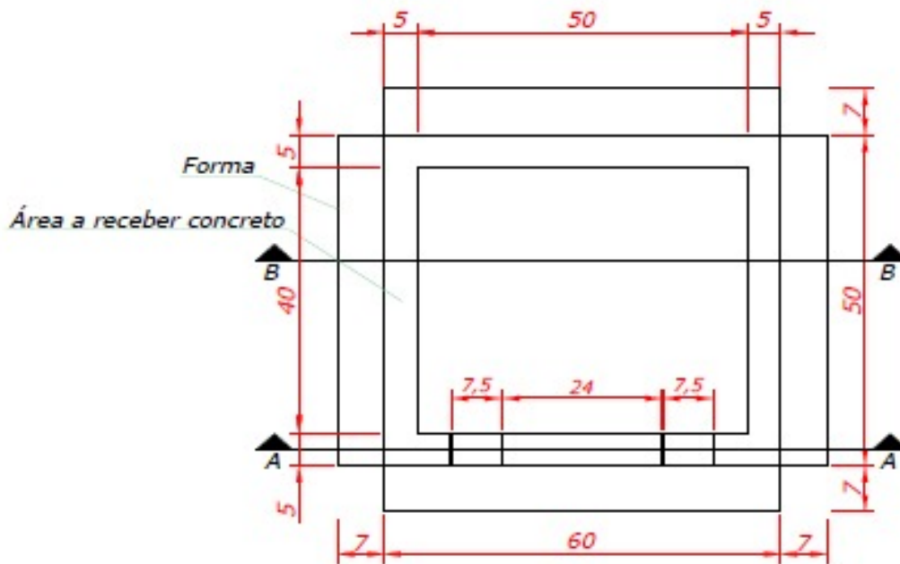
VISTA SUPERIOR
